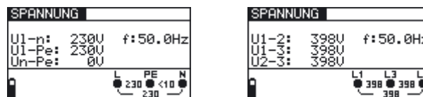
Abb. 5.41: Beispiele für Spannungs- und Frequenzmessung
