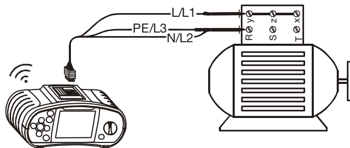
Abb. 5.10: Anschluss des Universalprüfkabels
